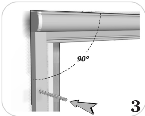
Position ermitteln / Befestigen der Seitenschiene durch Schrauben oder Kleben
